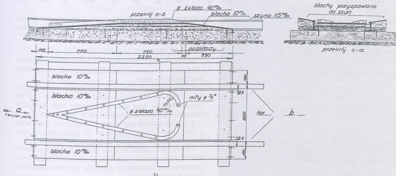
Wstawiacz wozów kop. na szyny kolejowe podczas biegu pociągu Podziałka 1:10
