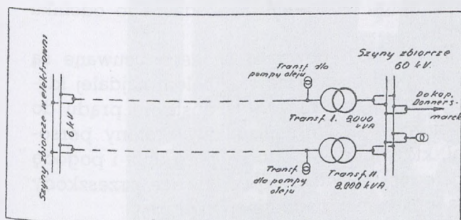
Ryc. 12. Schemat stacji transformatorowej 6/60 kV na kop. »Charlotte«.
