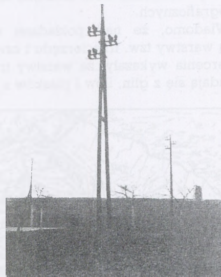
Ryc. 9. Skrzyżowanie szosy Wodzisław—Pszów przewodem 20 kV na słupach drewnianych i wsporczych izolatorach.
