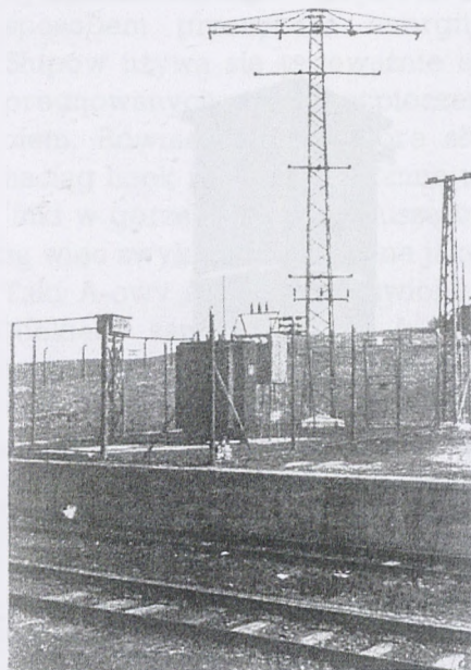
Ryc. 16. Napowietrzna stacja transformatorowa na szybie pow. III kop. »Anna«.
