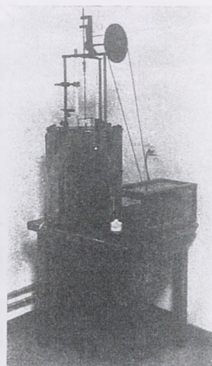
Kalorymetr określający wartość opałową węgla i koksu.
