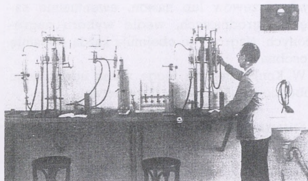
Aparaty służące do analizy gazów. Przy pracy laborant Szeja J.
