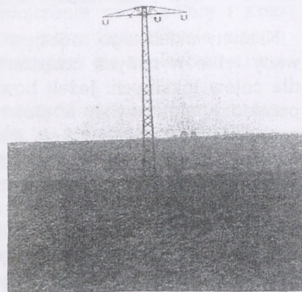
Ryc. 4. Przewód napowietrzny 20 kV »Anna—Ema« na słupach stalowych i wiszących izolatorach.
