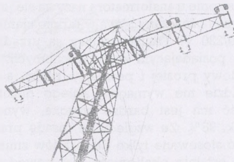
Ryc. 5. Głowica odporowego słupa stalowego z wiszącymi izolatorami. Szyb Jedłownik.
