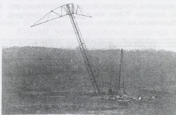
Ryc. 8. Stawianie słupa przelotowego przewodu napowietrzego 20 kV do szybu Jedłownik.
