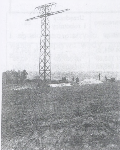
Ryc. 7. Słup odporowo-naróżny przewodu napowietrzego 20 kV do szybu Jedłownik, bezpośrednio po ustawieniu.
